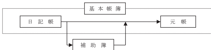
図表-2 ジョーンズの簿記の体系
