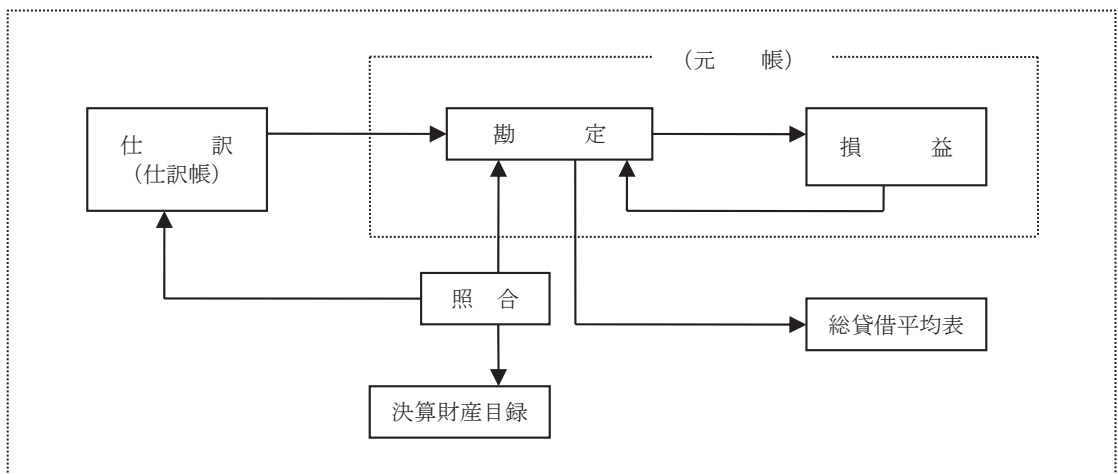
図表-1 マイスナーのイタリア式簿記による決算
